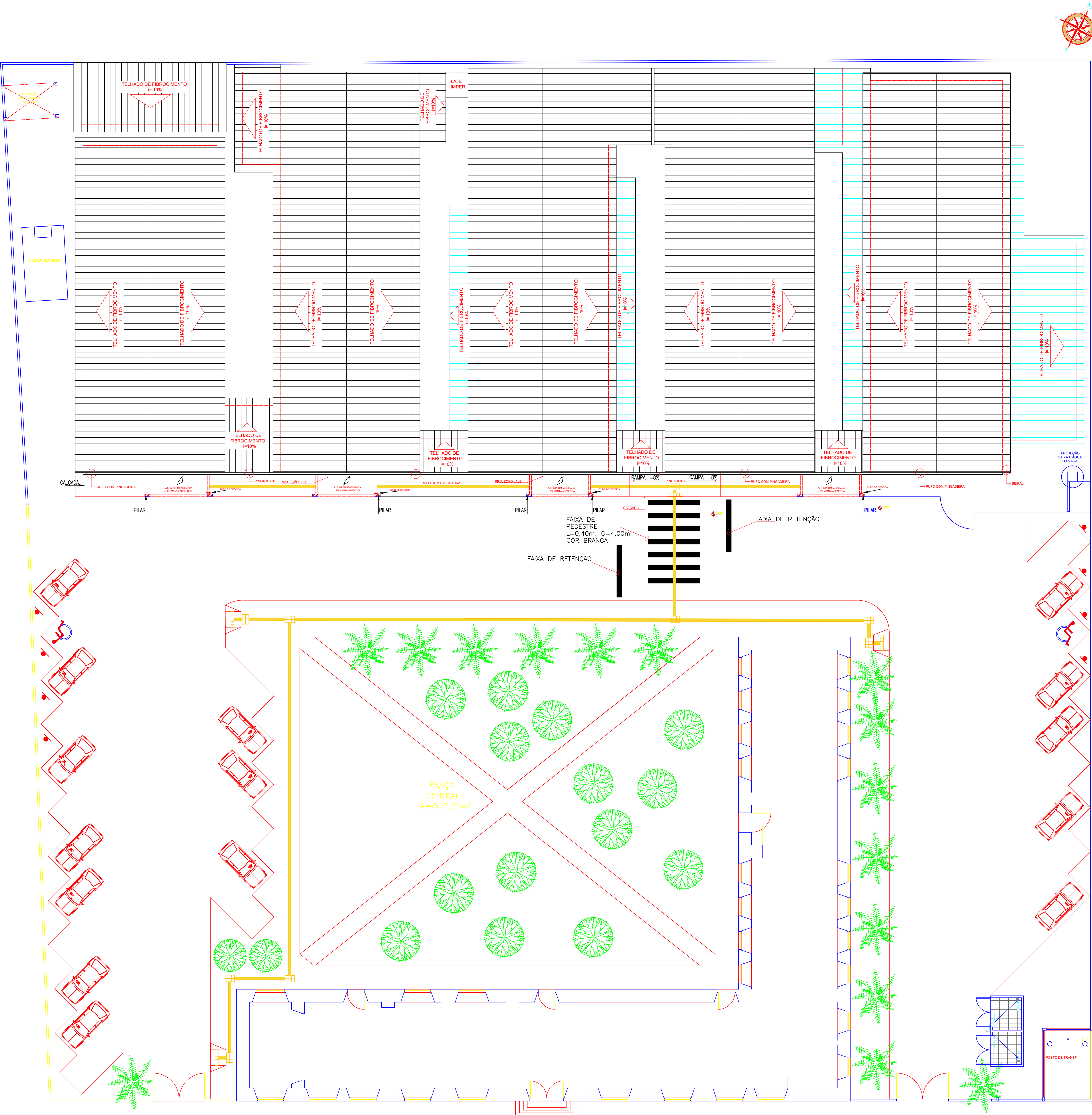
PLANTA DE IMPLANTAÇÃO esc. 1:125
